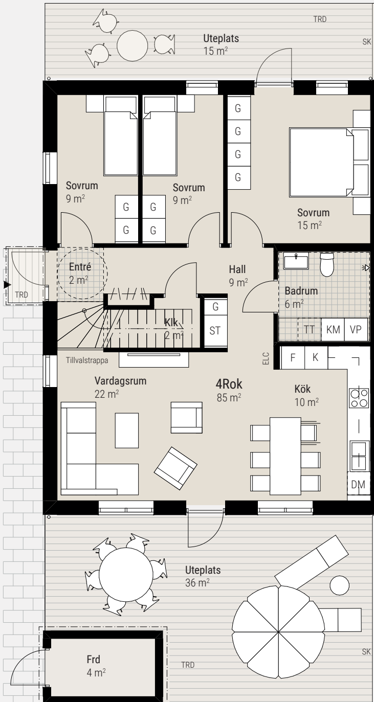
Nedre plan
