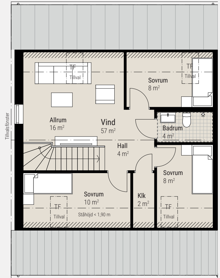
Övre plan
