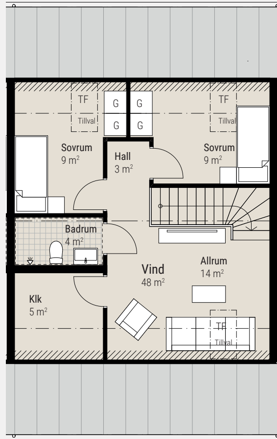
Övre plan
