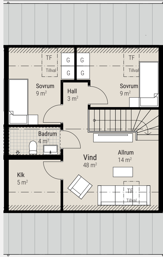
Övre plan
