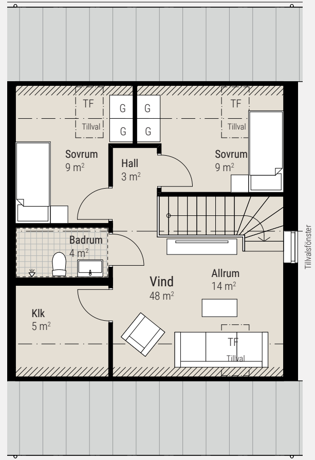
Övre plan
